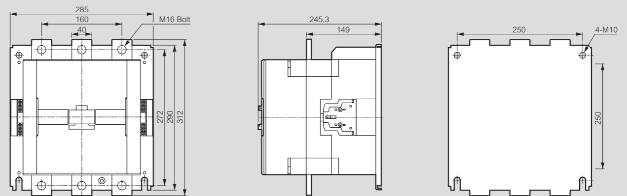
CTX 3 800
