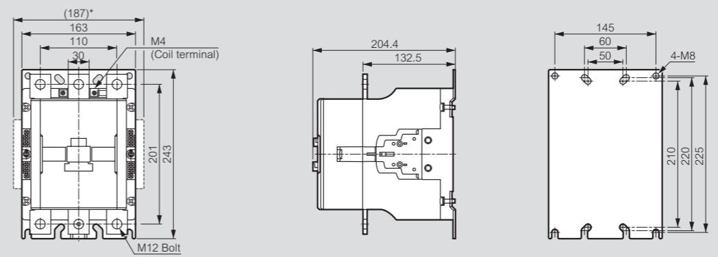
CTX 3 400
