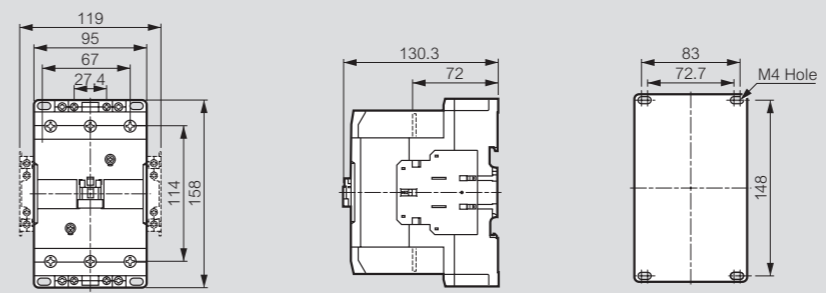
CTX 3 150
